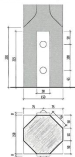
DET. B: UKONČENÍ U TERÉNU / M1:5
