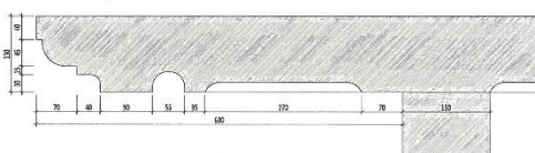
DET. A: ZHLAVÍ TRÁMŮ / M1:5
