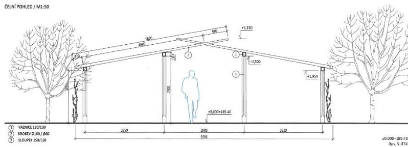
BOČNÍ POHLED / M1:50
